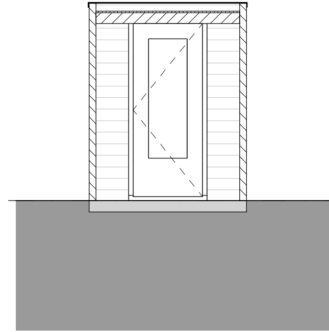
Doorsnede
