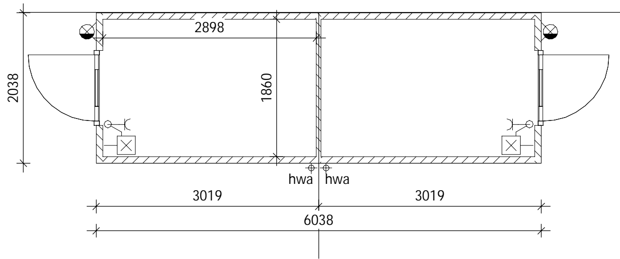
Plattegrond
